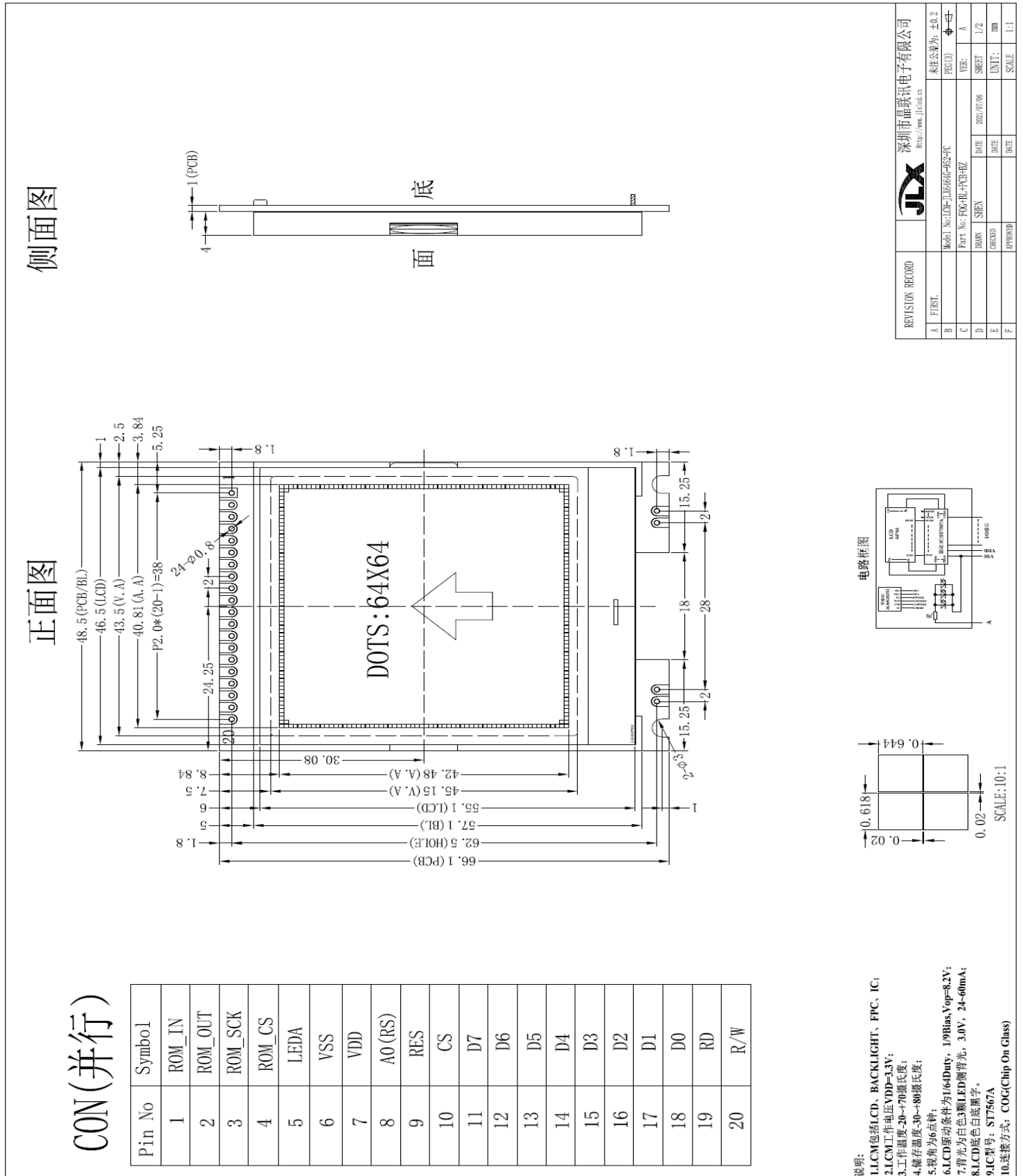
图 1. 外形尺寸
