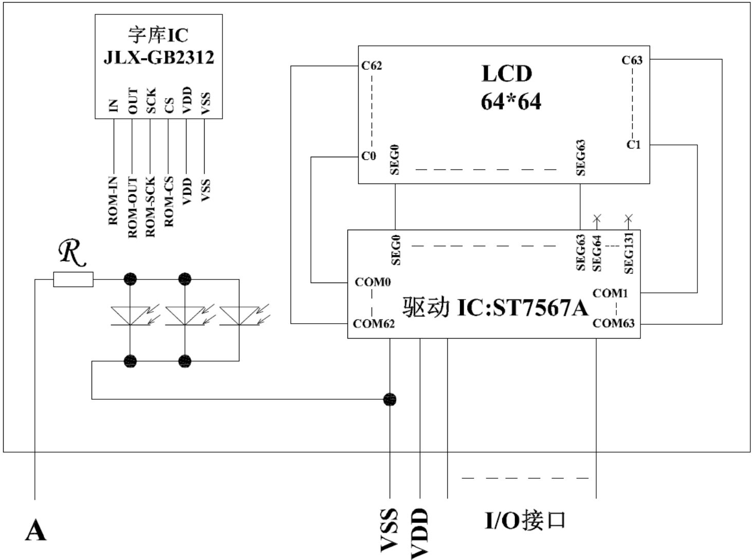
图 2: JLX6464G-952 图像点阵型液晶模块的电路框图
